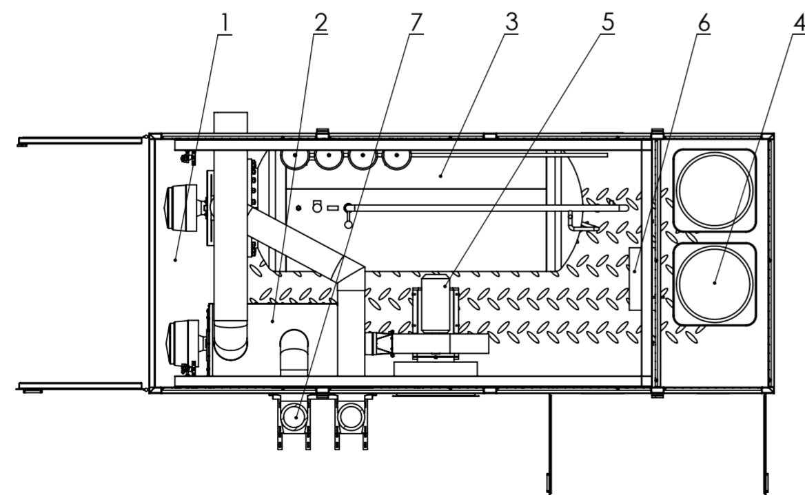
SEKTION A-A
